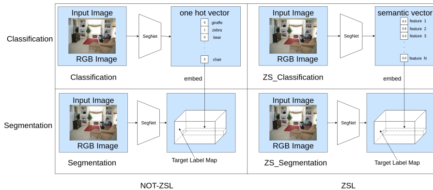
図1 物体認識の手法と ZSL の関係
