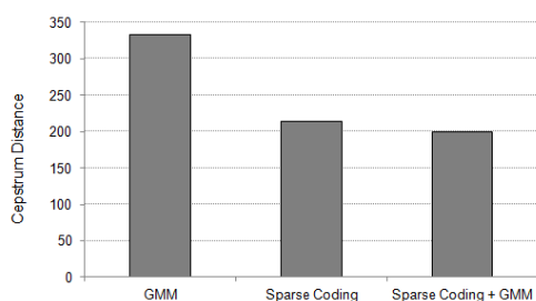
Fig. 4 目標音声と声質変換音声のケプストラム距離
