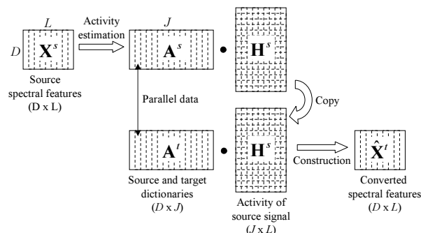
Fig. 1 Sparse Coding による声質変換の概要
