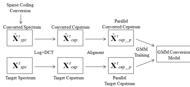
Fig. 3 変換後の特徴量を用いた GMM 学習の流れ
