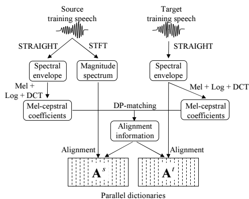
Fig. 2 パラレル辞書の構築
