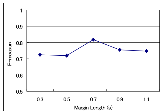
図5 マージンの長さシステム要求判別精度
