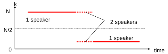
図7 CSP係数によるピークの現れ方 Fig. 7 CSP Peak Trace
