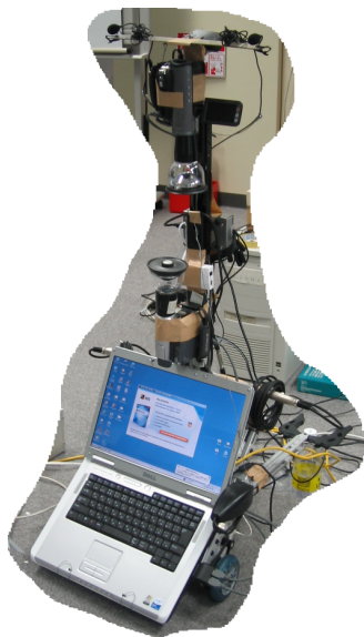
図2 本研究で用いたロボット Fig. 2 An image of the robot.
