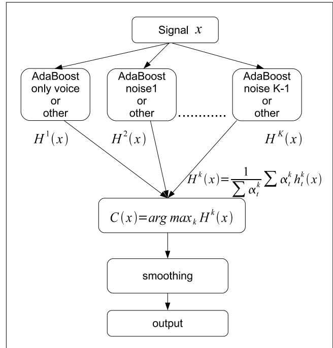
図 4 提案手法の概要
