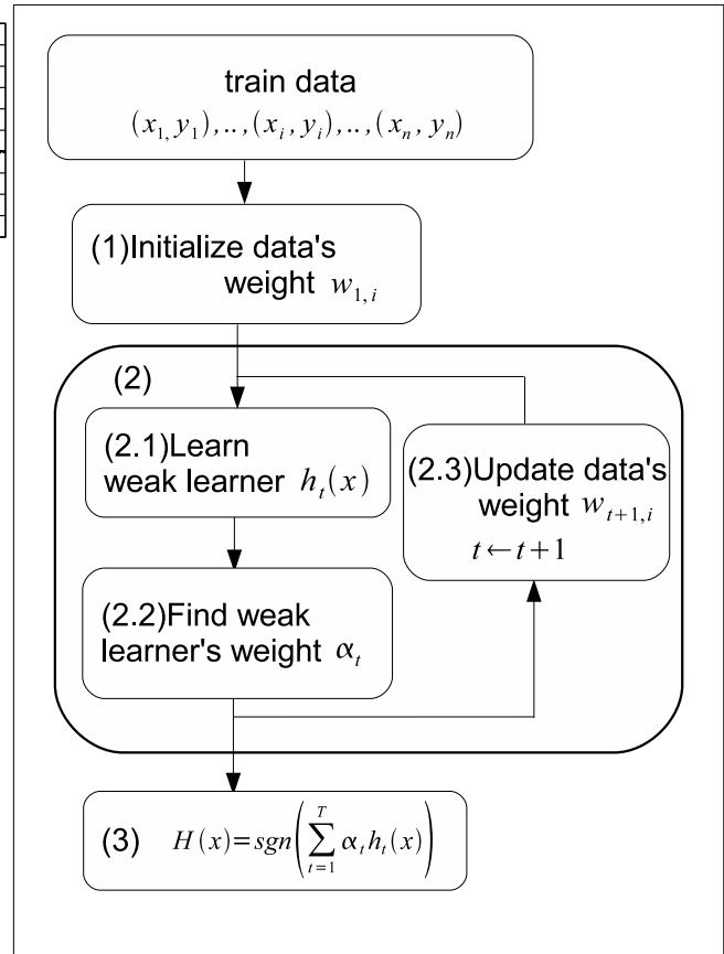
図3 AdaBoost の概要
