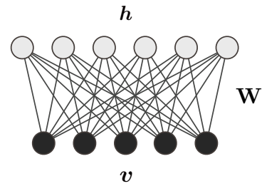
図 1 RBM のグラフ構造。
