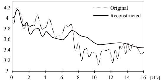
図5 入力話者の音声スペクトルと再構築されたスペクトル (上図), 出力話者の音声スペクトルと入力話者から出力話者へ変換されたスペクトル (下図).
