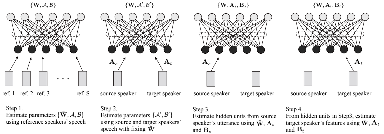
図3 適応型 RBM を用いた声質変換の流れ。
